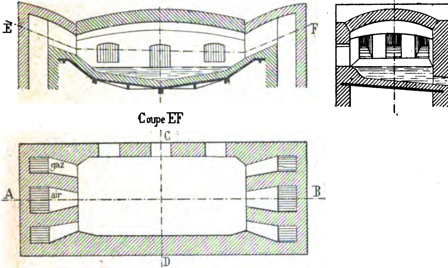
Fig. 137 à 139. — Four Siemens à voûte torseée.
